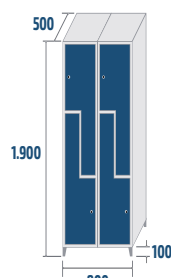
SL2-40/2 COD: 43045 44kg · 0,76m 3
