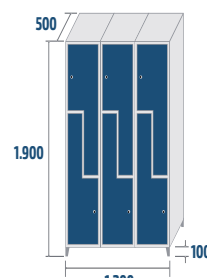
SL2-40/3 COD: 43145 63kg · 1,14m 3
