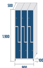
SL2-30/3 COD: 43043 53,1kg · 0,86m 3
