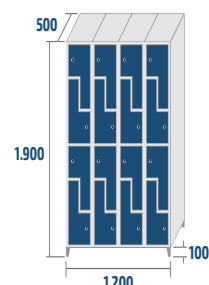
SL4-30/4 COD: 43153 69,1kg · 1,14m 3
