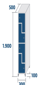
SL4-30/1 COD: 43051 21kg · 0,29m 3
