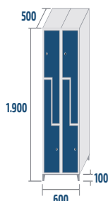
SL2-30/2 COD: 43042 37,1kg · 0,57m 3
