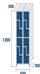
SL4-30/2 COD: 43052 37,1kg · 0,57m 3
