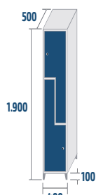
SL2-40/1 COD: 43044 25kg · 0,38m 3
