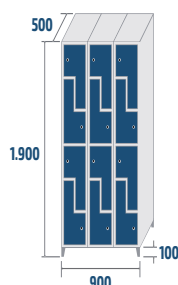
SL4-30/3 COD: 43053 53,1kg · 0,86m 3
