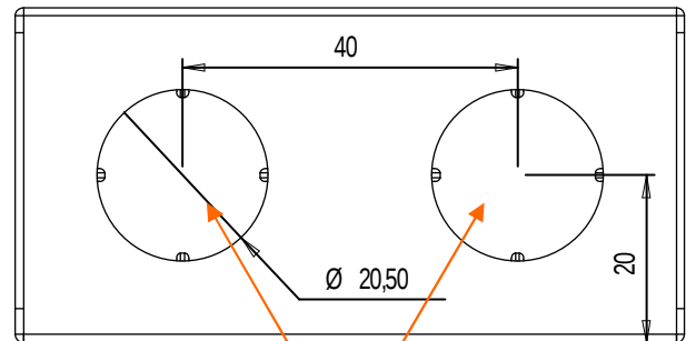
Boitier carré vue de dessous Beneath view of square casing model Untereansicht des viereckigen Gehäuse Vierkantige doos standpunt van onderkant
