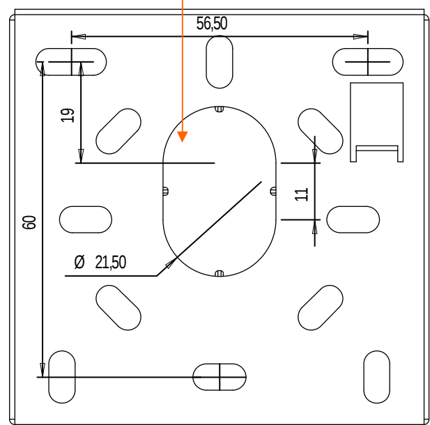
Boitier carré vue de dos Backside view of square casing model Hintereansicht des viereckigen Gehäuse Vierkantige doos standpunt achteraan
