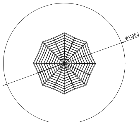
PT901 E: 1/200
