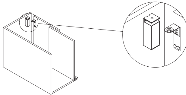
CONTREPARTIE STRIKE PLATE GEGENSTÜCK TEGENDEEL
