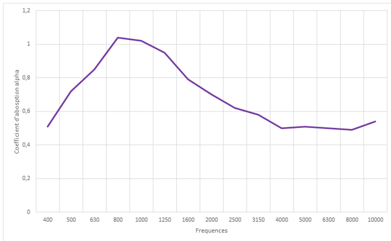
Indice d'absorption acoustique alpha
